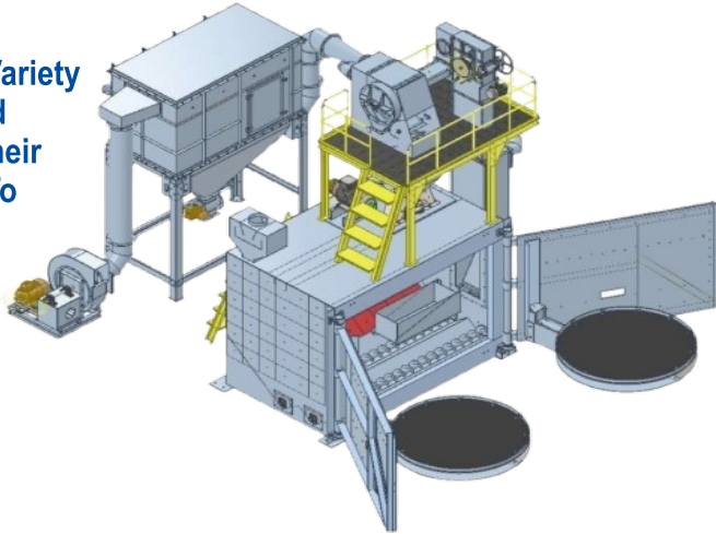
1800 DOUBLE DOOR SWING TABLE MACHINE
